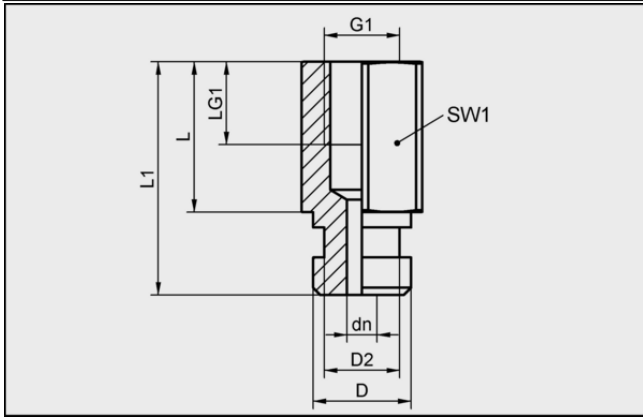
Tasarım verileri SA-NIP N021 M5-IG DN200
