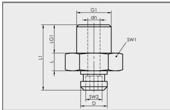
デザインデータ SA-NIP N022 G1/8-AG DN350
