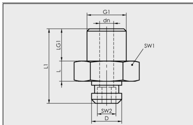
Конструктивные данные SA-NIP N022 G1/8-AG DN350
