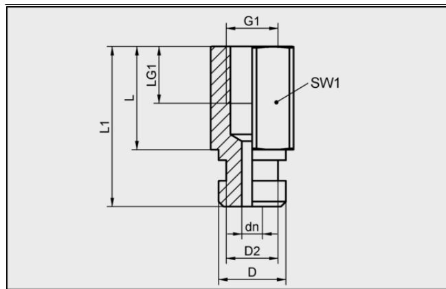
デザインデータ SA-NIP N022 G1/8-IG DN350
