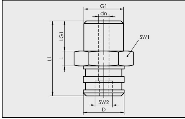
Tasarım verileri SA-NIP N023 G1/4-AG DN350
