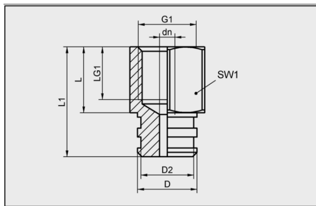
Конструктивные данные SA-NIP N023 G1/4-IG DN350
