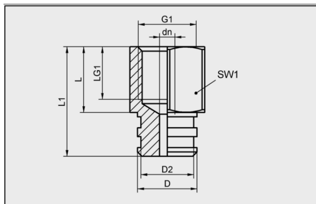
デザインデータ SA-NIP N023 G1/4-IG DN350
