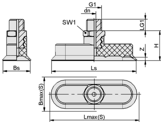
デザインデータ SGON 15x5 NBR-55 M5-AG
