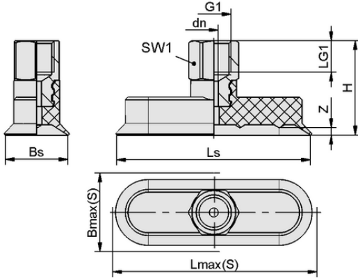
Tasarım verileri SGON 15x5 NBR-55 M5-IG
