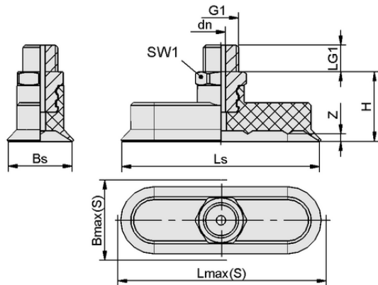
デザインデータ SGON 24x8 NBR-55 G1/8-AG
