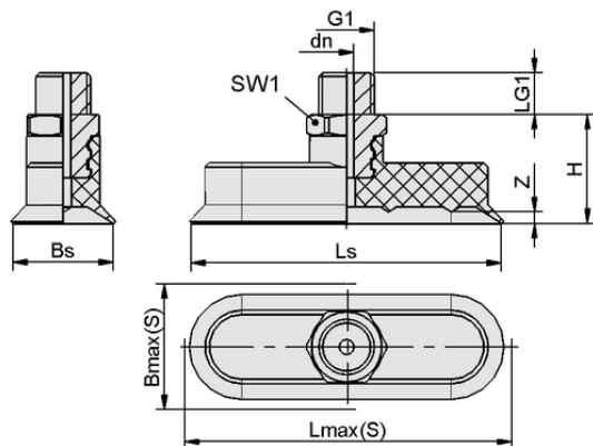
デザインデータ SGON 30x10 NBR-55 G1/8-AG
