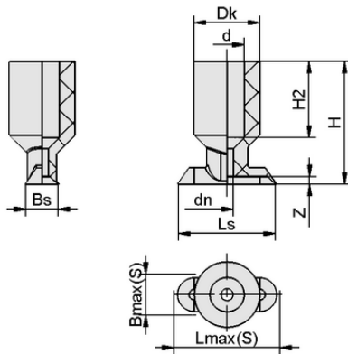
Datos de diseño SGO 15x5 NBR-55 N021
