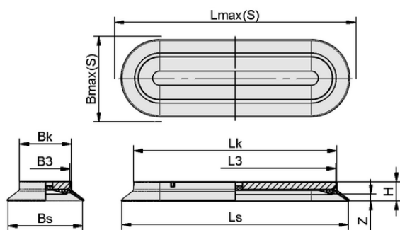
Конструктивные данные SPLO 200x55 NBR-55
