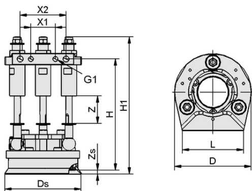
Конструктивные данные DBD 130x187 80 M54
