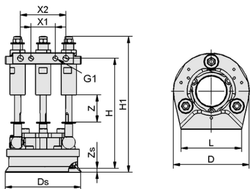
Конструктивные данные DBD 100x189 80 M42
