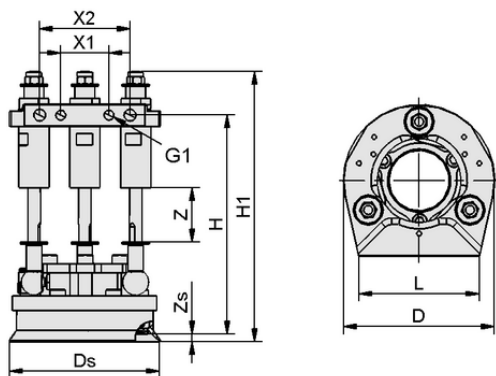
Données de construction DBD 100x189 80 M42
