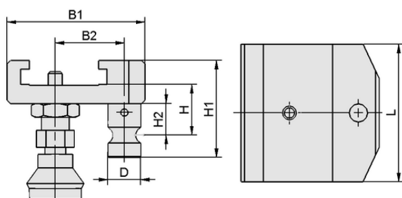
Конструктивные данные HTS-A2 DBD QC1-A
