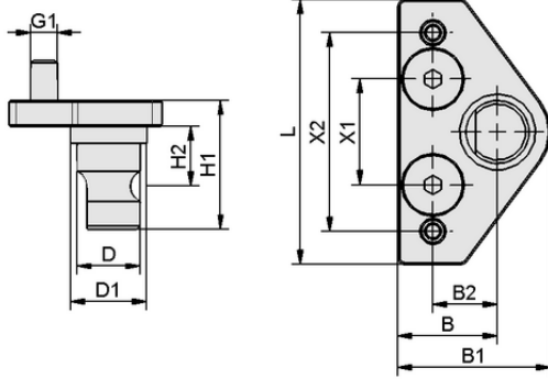
Tasarım verileri HTS-A2 DBD
