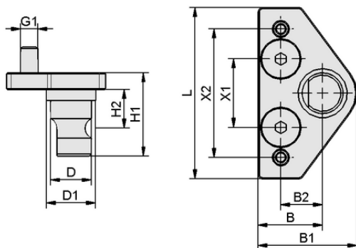
Конструктивные данные HTS-A2 DBD
