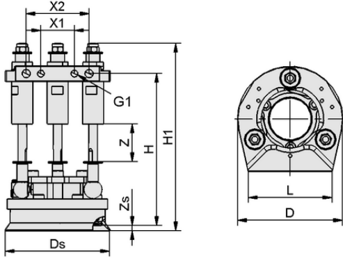
Tasarım verileri DBD 100x145 36 M42
