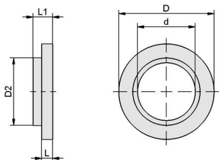
デザインデータ SCHE 38-18.5x5 ST VZ
