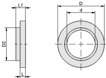
Konstruktionsdaten SCHE 38-18.5x5 ST VZ
