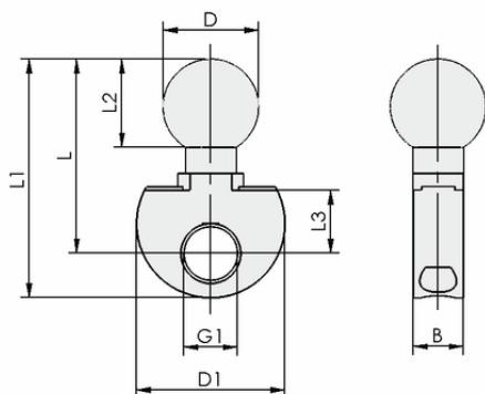
Dati di costruzione HTR-FST A3 FSTI
