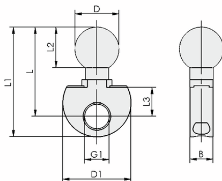
Конструктивные данные HTR-FST A3 FSTI
