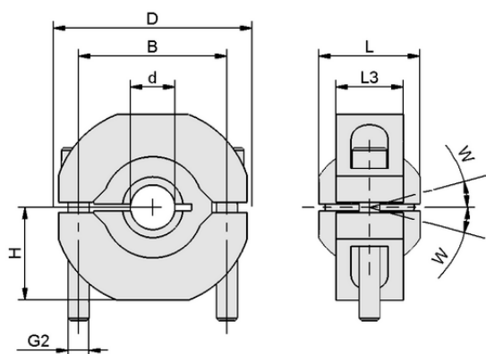
Конструктивные данные HTR-UNI 2N FSTE-HDB
