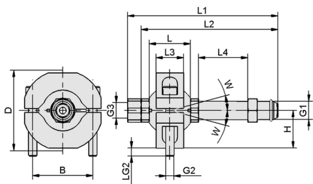
Конструктивные данные HTR-UNI 2N G2 110
