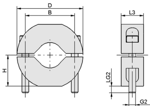
Конструктивные данные HTR-UNI 2N X3
