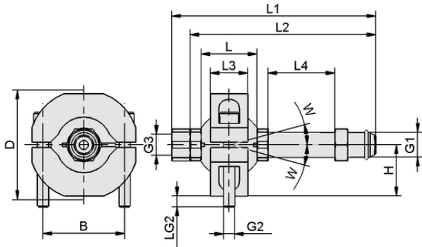
Tasarım verileri HTR-UNI 2N G2 140
