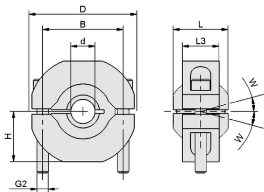
Конструктивные данные HTR-UNI 2N G1/4
