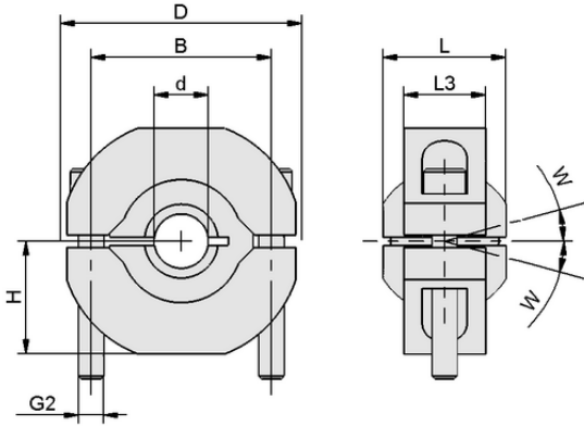
Tasarım verileri HTR-UNI 2N G1/4
