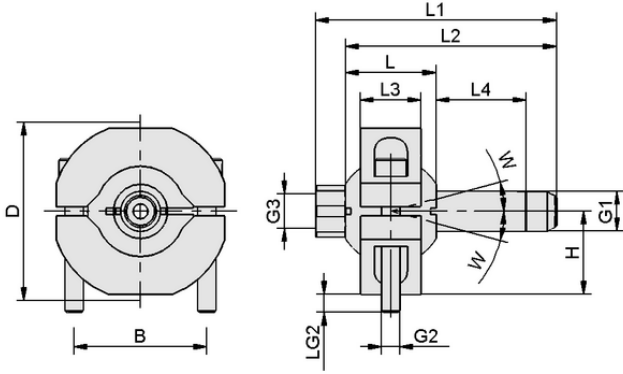
Tasarım verileri HTR-UNI 2N G2 80
