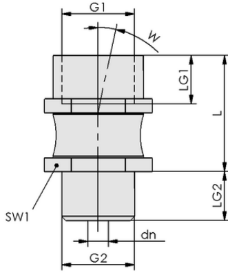
Tasarım verileri FLK G1/2-IG G1/2-AG V
