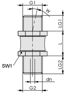
Tasarım verileri FLK G1/2-AG G1/2-AG
