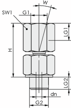
Tasarım verileri KGL G1/4-IG M10x1.25-AG
