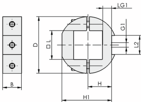
Konstruktionsdaten HTR-STB 30x30 UNI
