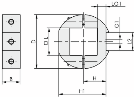
Tasarım verileri HTR-STB 30x30 UNI
