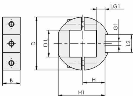
Datos de diseño HTR-STB 30x30 UNI
