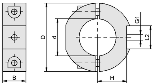
Konstruktionsdaten HTR-STC D32 UNI
