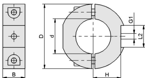
デザインデータ HTR-STC D32 UNI
