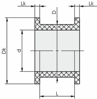
Tasarım verileri BUCHSE 32-25x21 PA
