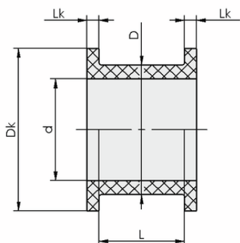
Конструктивные данные BUCHSE 32-25x21 PA
