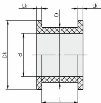
Konstruktionsdaten BUCHSE 32-25x21 PA
