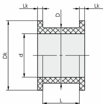
Données de construction BUCHSE 32-25x21 PA
