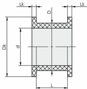
Datos de diseño BUCHSE 32-25x21 PA
