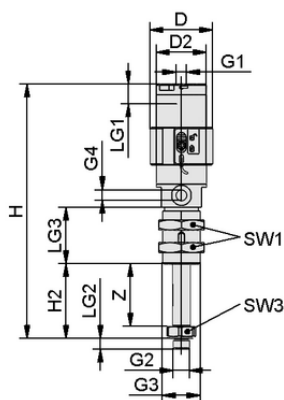
Конструктивные данные FST-LOCK-HD G1/4-AG 100 NC VG SFP
