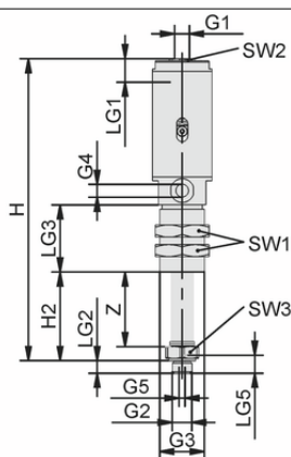
Конструктивные данные FST-LOCK-HD G1/4-AG 100 NC AB
