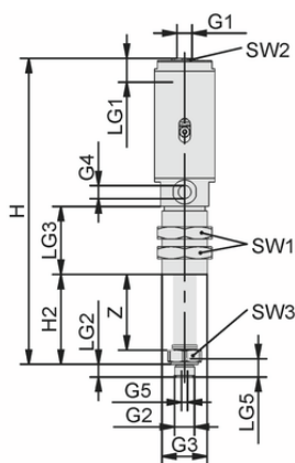
デザインデータ FST-LOCK-HD G1/4-AG 50 NC AB
