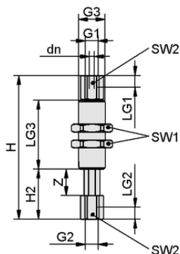
デザインデータ FSTIm M5-IG M5-IG A 5 VG-IN
