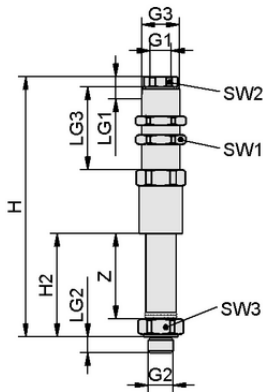
Design data FSTE-HDB G3/8-AG 25 VG-AB
