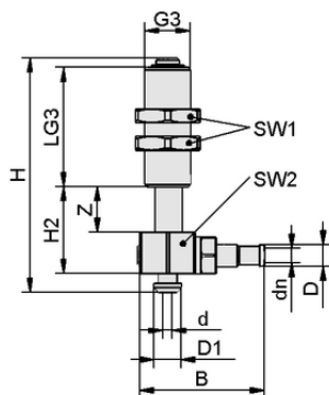
Конструктивные данные FSTIm N004 6/4 L 10 IN
